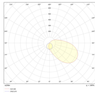
Tuscan G2 60 Polar Curve
